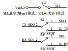
在SEL跳线时, 同时也需要跳TX_SDO, RX_SDI
