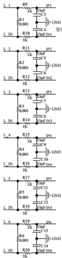
R1~R6电流采样电阻精度要求1%以上 50ppm R9-R20电阻1K 0.1% 25ppm
