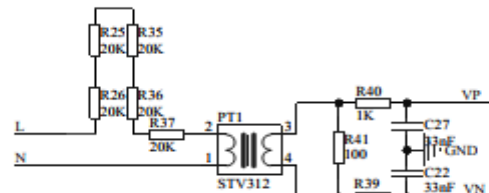
电压互感器1:1, 2mA, 负载电阻采用100欧, 220V电压时VP管脚电压220mV 电压通道PGA增益1倍 20K分压电阻精度0.5%以上, PT电压互感器, 批量一致性0.5%以上, R46负载电阻精度0.5%以上
