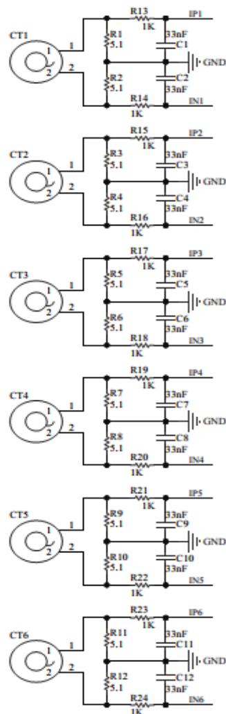
电流互感器2000:1,最大电流30A; 负载电阻5.1欧*2, IP, IN最大信号=30A*5.1欧*2/2000=153mV 电流通道PGA增益可以用2倍 5.1欧负载电阻精度0.5%以上; CT1~CT6电流互感器, 批量一致性要求0.5%以上
