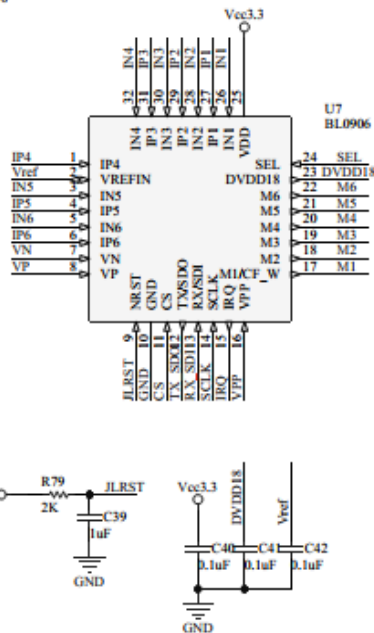
M1可复用为电能脉冲输出管脚
