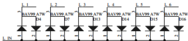
保护电路, 根据需要添加
